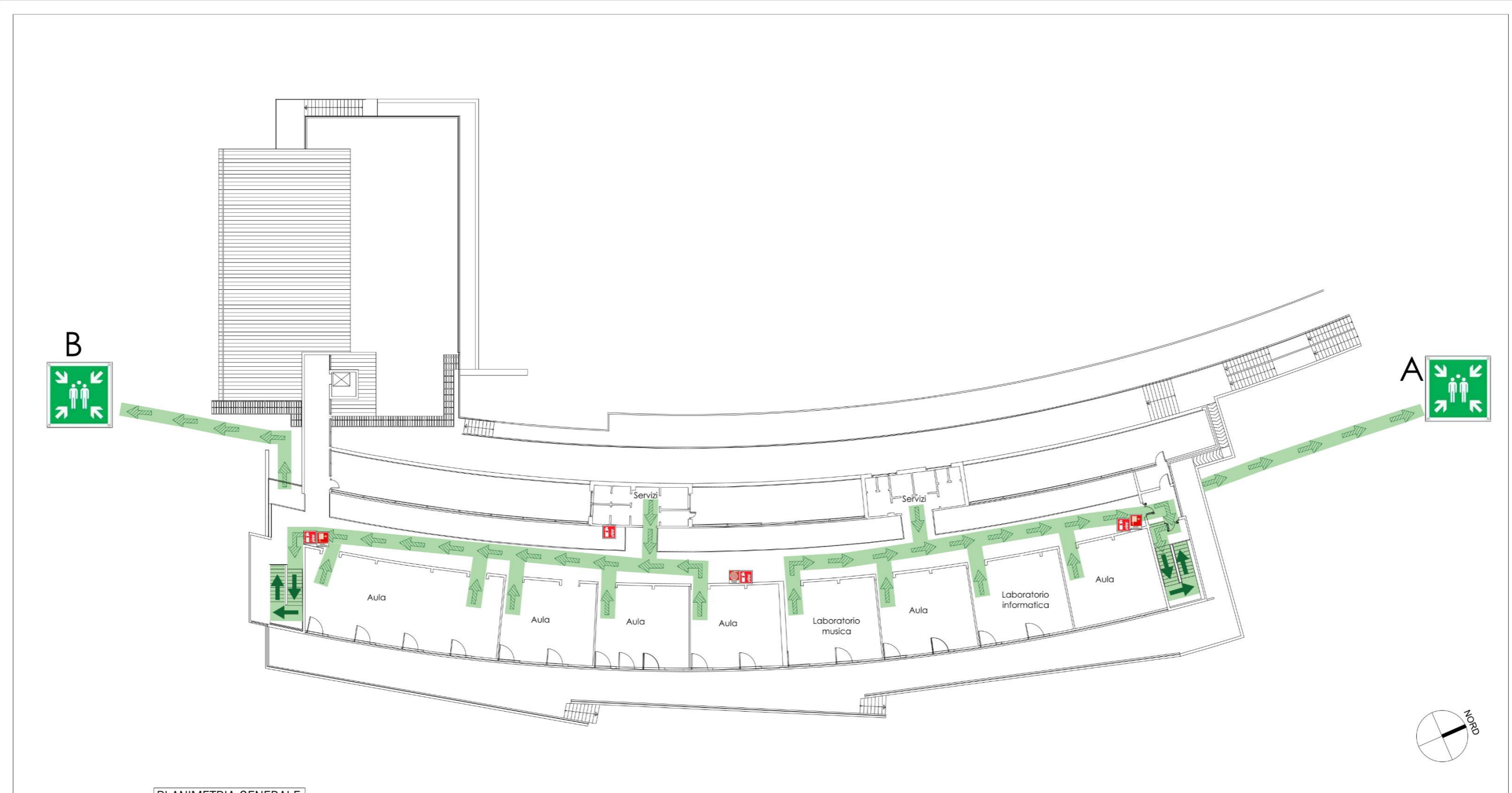
PLANIMETRIA GENERALE
